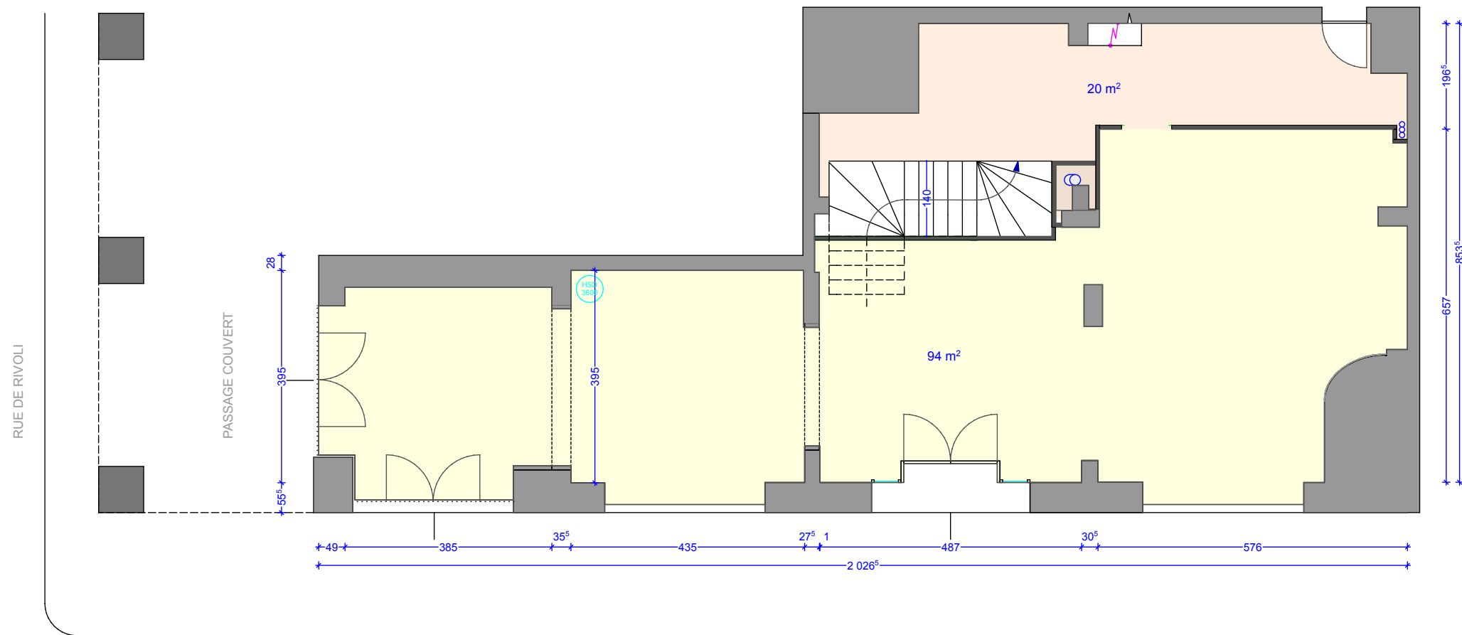
PLAN REZ DE CHAUSSEE EXISTANT
